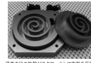
渦巻状の旋盤がスクロールして空気を圧縮
